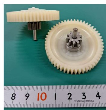
〈電動パーキングブレーキ構成部品〉 特徴: インサートモールド品
